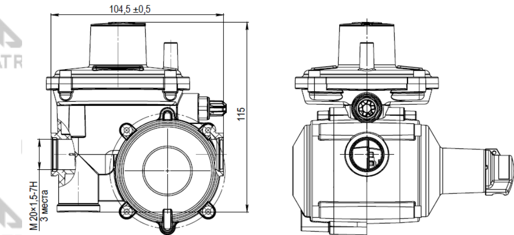
РИСУНОК 3. ГАБАРИТНО-МОНТАЖНЫЕ РАЗМЕРЫ
